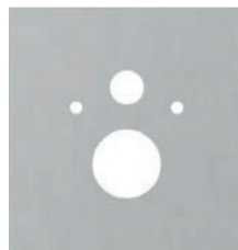
Standartinis unitazas Art.Nr. 9 650 100 TECEone Art.Nr. 9650109 Standartinis unitazas Art.Nr. 9 650 105 TECEone Art.Nr. 9650110
